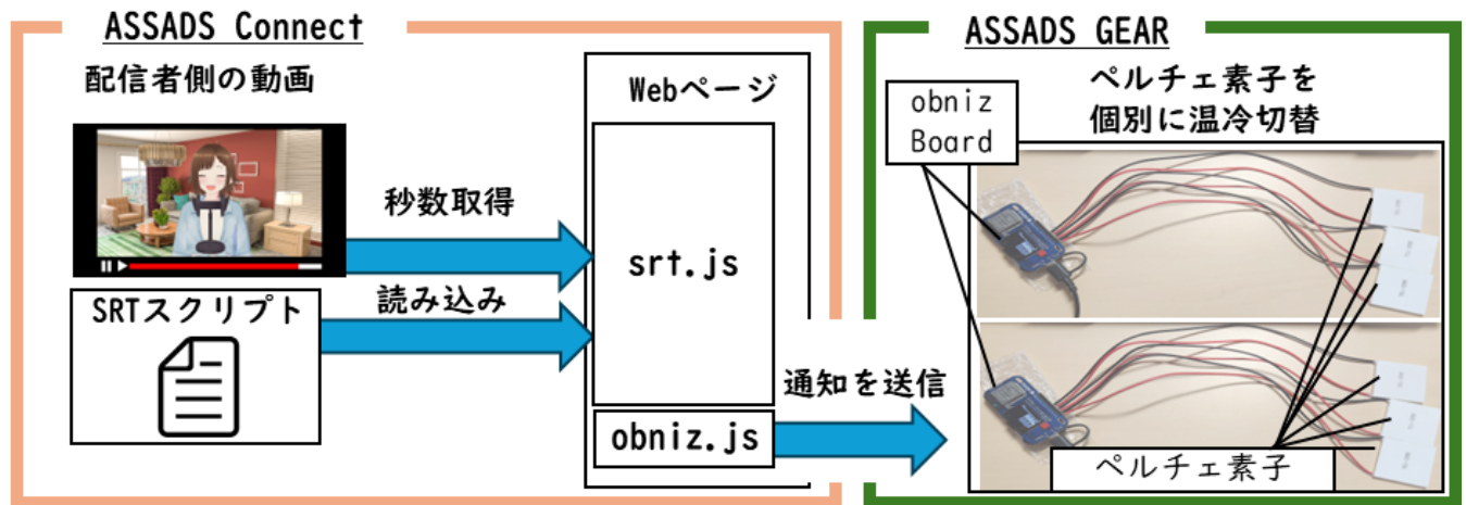
図 1: ASSADS システム構成
